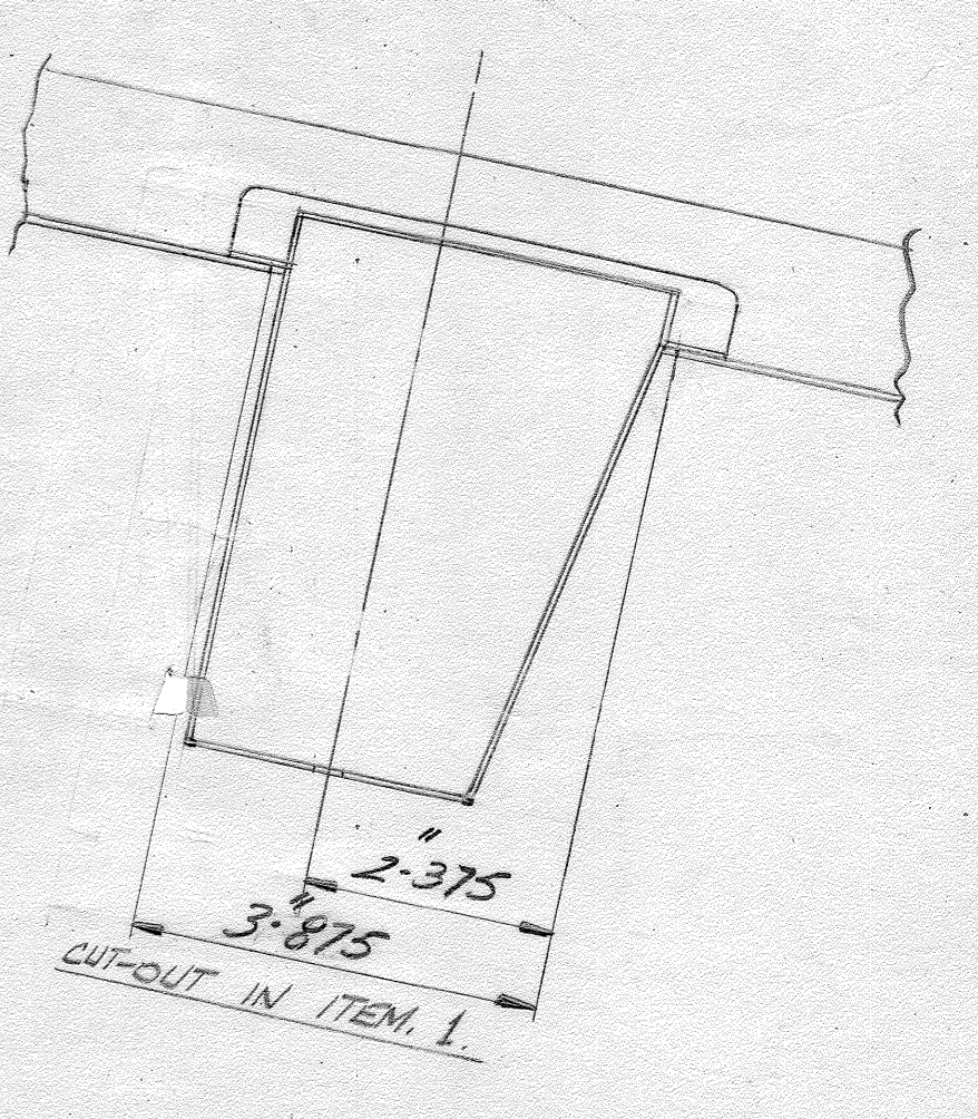
SECTION 'B-B'
